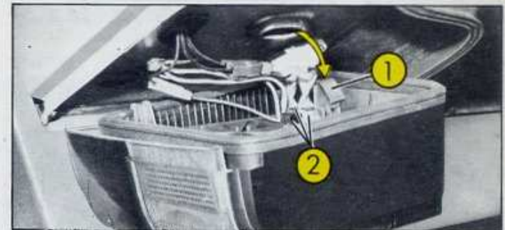
Fig. 7 Boîtier de signalisation arrière 1 - Ressort de maintien 2 - Connecteurs
