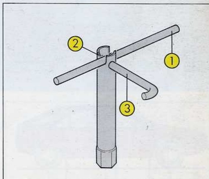
Fig. 12 Bougies
