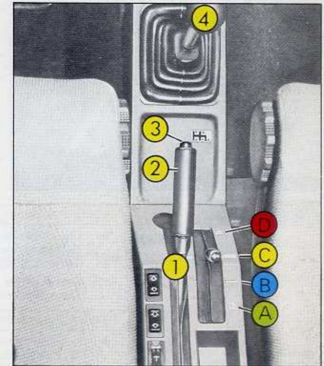
Fig. 18 1 - Réglage de garde au sol 2 - Frein de secours et d'immobilisation 3 - Bouton de déverrouillage 4 - Levier de vitesses
