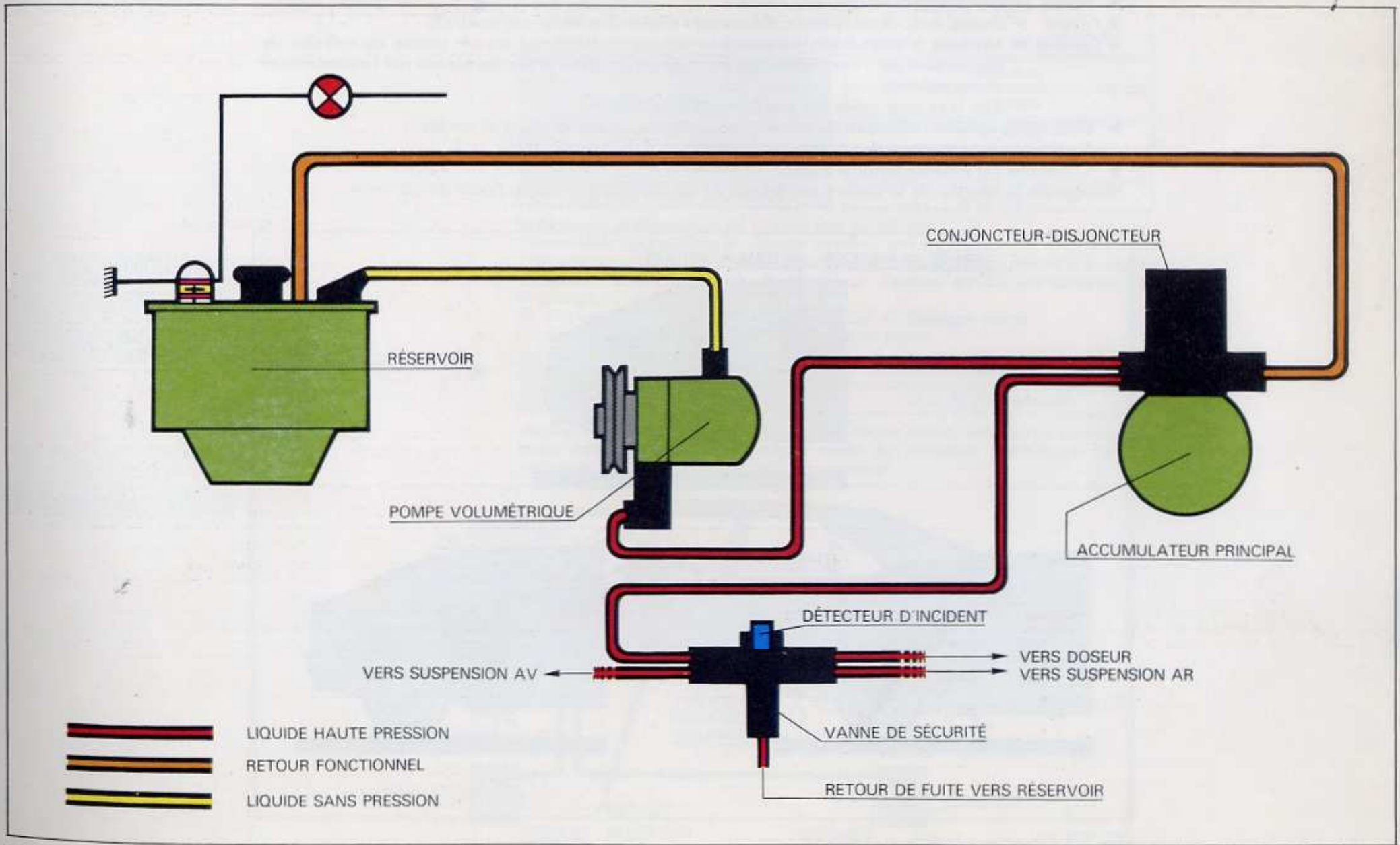
Fig. 2 Réserve de pression hydraulique
