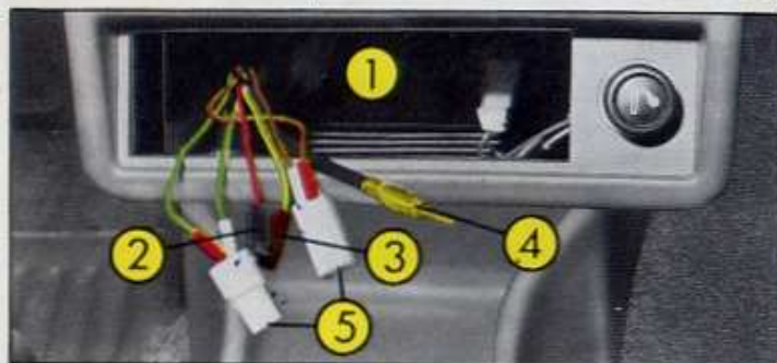
Fig. 7 Branchement auto-radio 1 - Emplacement du poste 2 - Alimentation auto-radio 3 - Masse auto-radio 4 - Coaxial d'antenne 5 - Connecteurs de haut-parleurs
