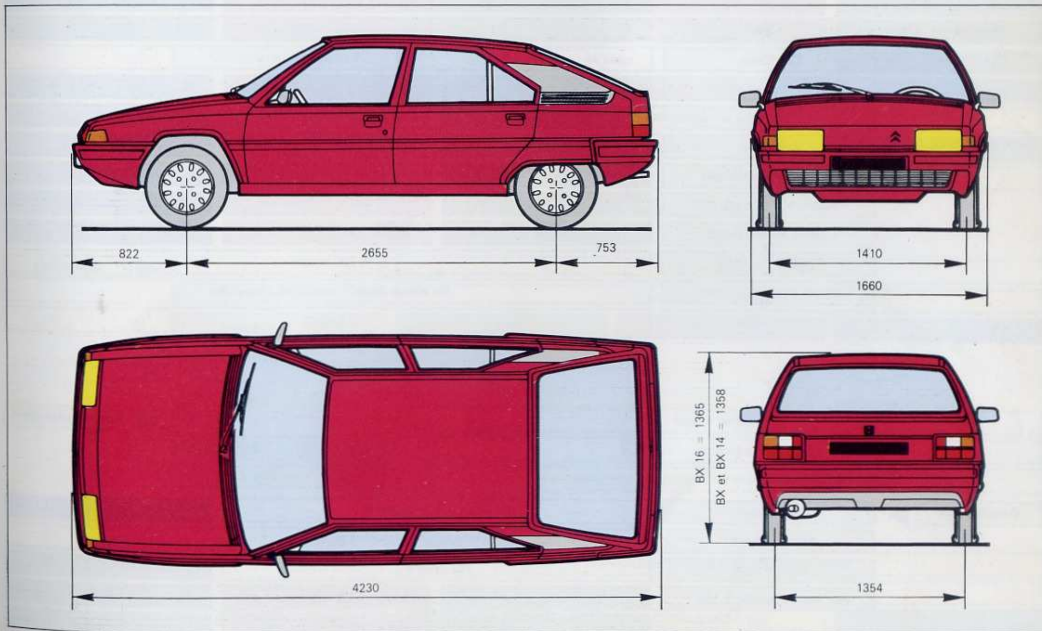
Fig. 1 Cotes d'encombrement
