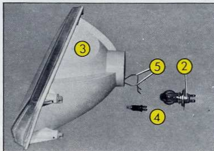
Fig. 5 Lampe de projecteur 2 - Colletette d'ampoule 3 - Parabole du projecteur 4 - Ampoule de lanterne 5 - Ressort de maintien
