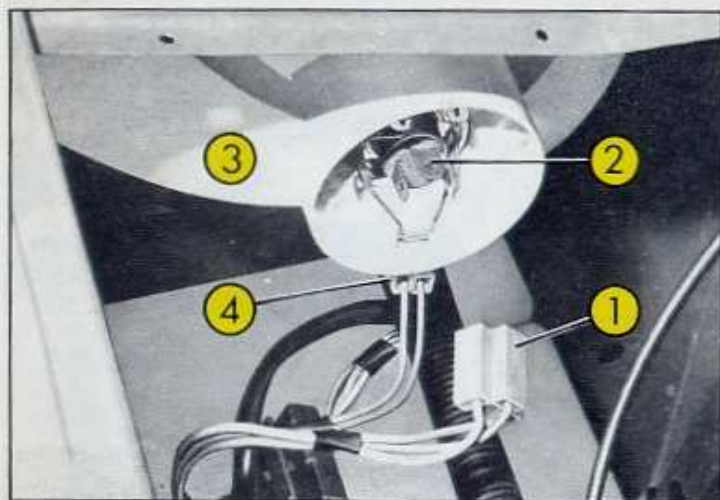
Fig. 3 Lampe de projecteur 1 - Connecteur 2 - Colletette d'ampoule 3 - Parabole du projecteur 4 - Lanterne
