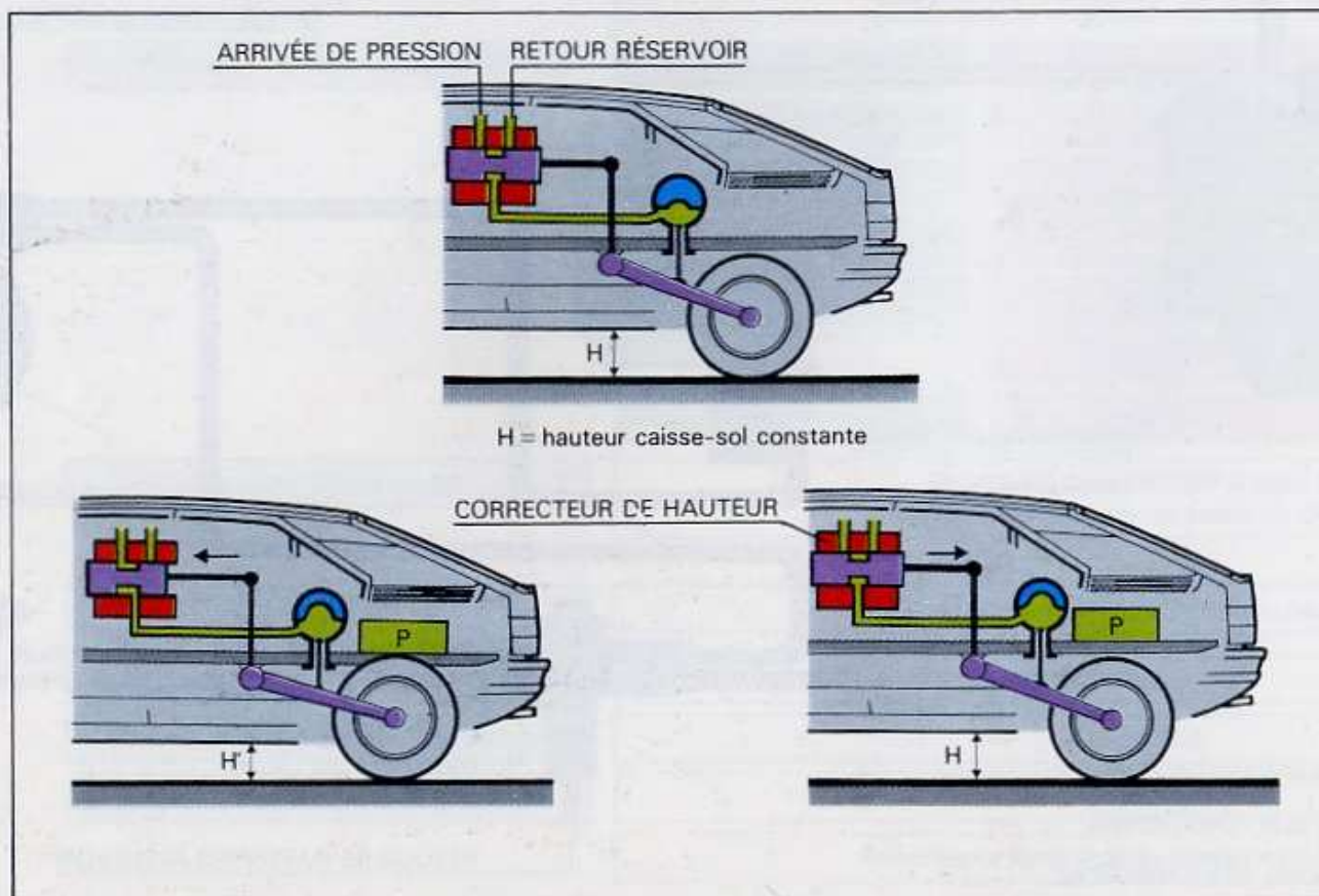
Fig. 3 Correction d'assiette
