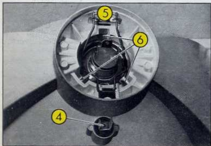
Fig. 4 Lampe de projecteur 4 - Lanterne 5 - Ressort de maintien 6 - Crans d'orientation de l'ampoule
