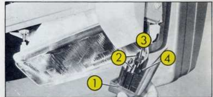
Fig. 6 Indicateurs de direction avant 1 - Boîtier 2 - Languettes d'accrochage 3 - Connecteur 4 - Porte-lampe
