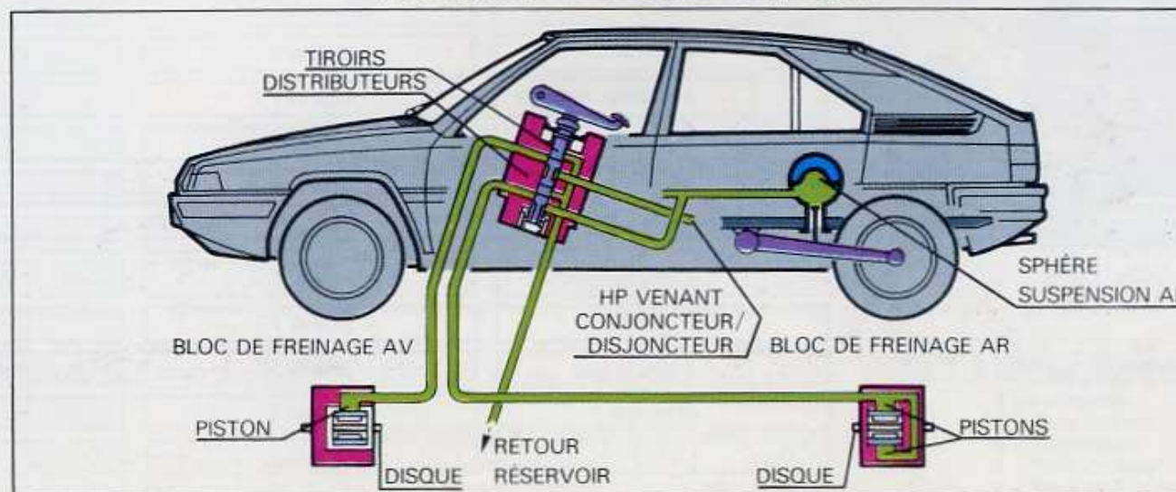
Fig. 4 Schéma de freinage
