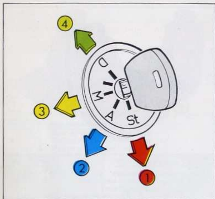
Fig. 15 Combiné « Antivol-Contact-Démarreur »
