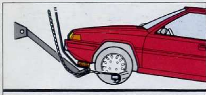
Fig. 13 Remorquage par l'avant
