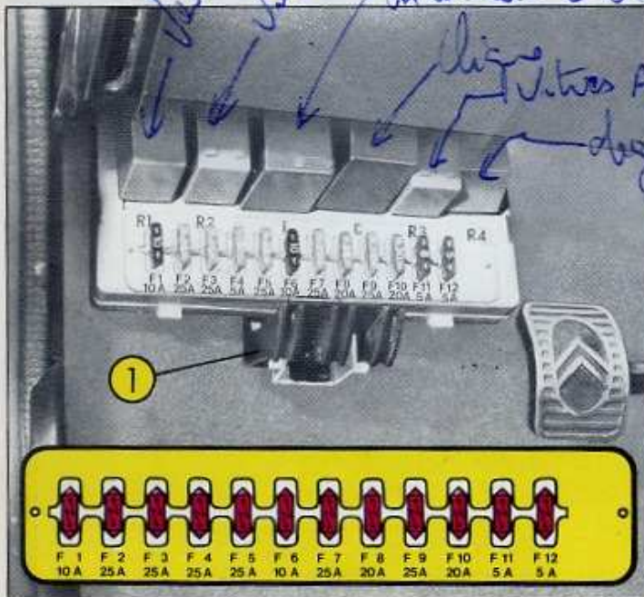
Fig. 10 Boîtier des fusibles 1 - Palette de déverrouillage
