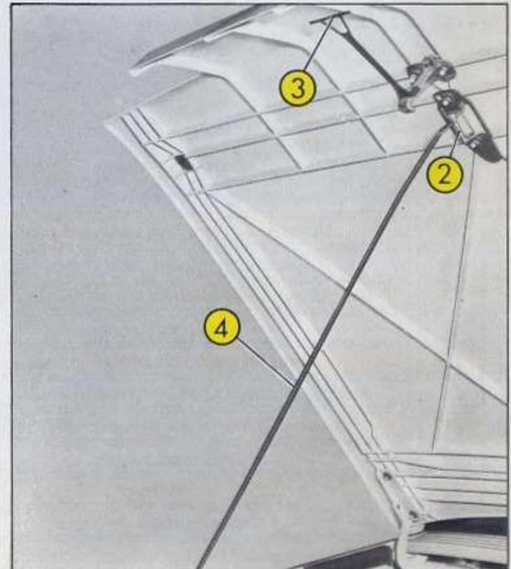
Fig. 5 Ouverture du capot 2 - Pêne de verrouillage 3 - Languette crochet de sécurité 4 - Béquille de maintien
