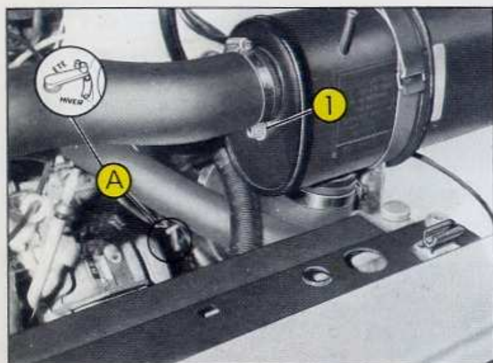
Fig. 3 Filtre à air
