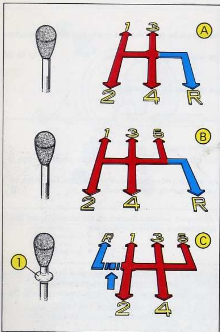
Fig. 17 Levier de vitesses
