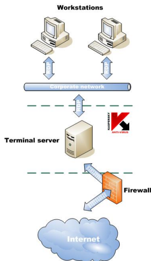
Illustration 3. Schéma de protection des serveurs de terminaux
